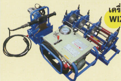
เครื่องควบคุมการเชื่อม WIZDOM DATA LOGGER
