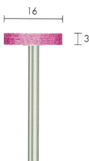
WS-1603 (16x3mm.)
