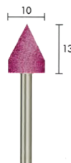
A-1013K (10x13mm.)
