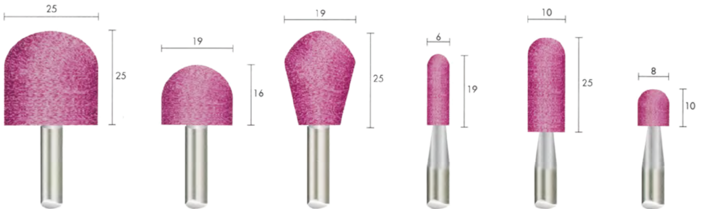
A-21 (25x25mm.)
