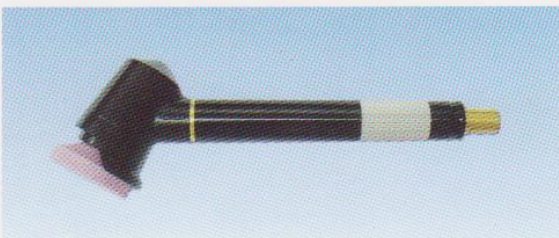
ความเร็วรอบ / Free Speed at 90 psi : 22,000 rpm หัวยึดเกี่ยวเชื่อม / Collet chuck : M7 screw shaft / M7 ขนาด / Dimensions : \varnothing 16.5 \times 136L (mm) น้ำหนัก / Weight : 200 g
