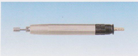
ความเร็วรอบ / Speed : 60,000 rpm น้ำหนัก / Weight : 130 g ขนาด / Dimensions : \varnothing 17 \times 159L (mm)
