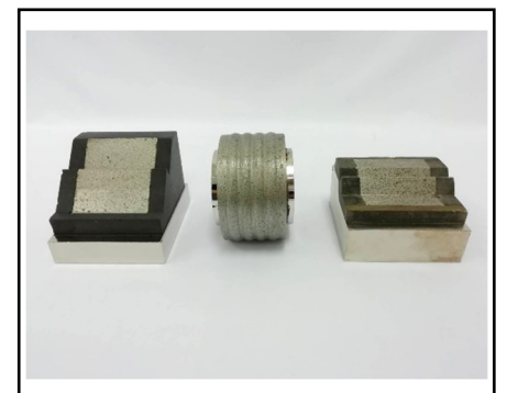
PRECISION REVERSE PLATING FORMED BLOCK & WHEEL หินเจียรชนิดชุบเพชรสำหรับงานพรีซิชัน ชนิด BLOCK
