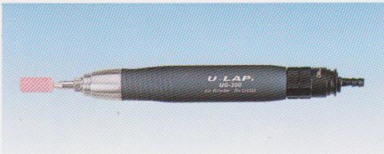
ความเร็วรอบ / Speed : 35,000 rpm น้ำหนัก / Weight : 170 g ขนาด / Dimensions : \varnothing 22 \times 180L (mm)
