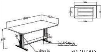
NIB-ALU1810 โต๊ะปฏิบัติการกลางแบบที่ 2
