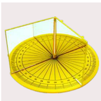
รหัส 21617 950.- / ชุด ชุดศึกษาการเกิดภาพบนกระจก (Pudak) Folding Flat Mirror (Pudak)
