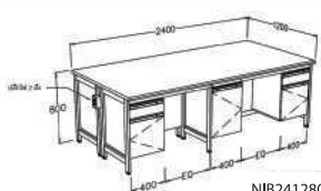
NIB241280 โต๊ะปฏิบัติการกลางแบบที่ 1
