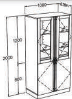
NTC105020 ตู้เก็บอุปกรณ์ แบบที่ 2
