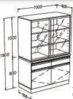
NTC106018 ตู้เก็บอุปกรณ์ แบบที่ 1
