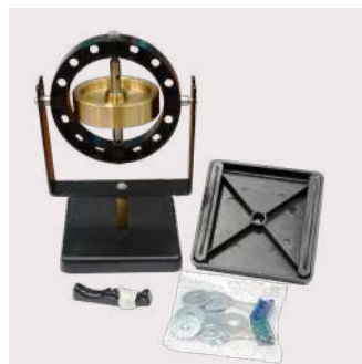
รหัส 21527 2,200.- / ชุด ไจโรสโคป Gyroscope ใช้ทดลองเกี่ยวกับโมเมนตัมเชิงมุม โดยอาศัย แรงเฉื่อยของล้อหมุน ขนาดอุปกรณ์ 100x100x175 มม.
