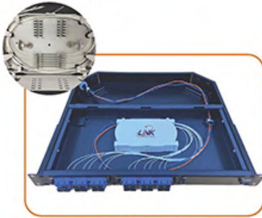
SP-2200 การต่อสายด้วยวิธี FUSION SPLICE
