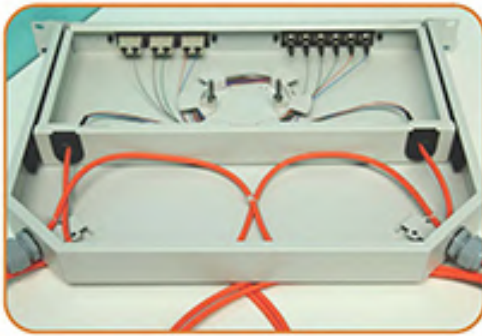
SP-2301 การติดตั้งแผงจัดสายอุปกรณ์ F.O. Drawer / FDU ขนาด 1 U
