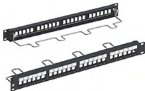
AMC-3620 SHIELDED 24P PATCH 1U, UNLOADED แผงต่อสาย 24 Port CAT 6A SHIELDED
