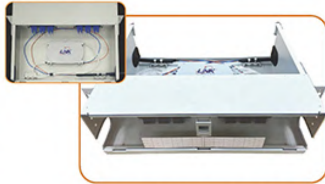
SP-2302 / SP-2303 / SP-2304 / SP-2306 การติดตั้งแผงจัดสายอุปกรณ์ F.O. Drawer / FDU ขนาด 2 U - 5 U
