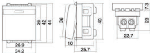
Figure 5 - สวิตช์ 2 ทางขนาดกลาง
