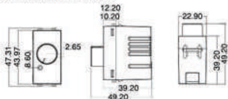
Figure 22 - สวิตช์ไฟหลอดไส้ ขนาดมาตรฐาน
