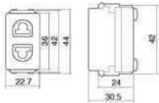
Figure 9 - ตัวรับคู่เสียบขากลมแบบ มีกราวด์
