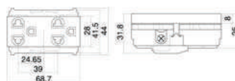
Figure 4 - ตัวรับเชื่อมต่อแบบขากรวย
