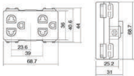
Figure 9 - ตัวรับคู่เสียบขากลมแบบ มีกราวด์
