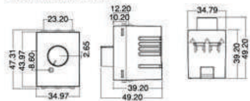
Figure 23 - สวิตช์ไฟหลอดไส้ ขนาดกลาง
