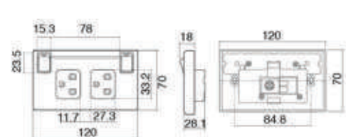
Figure 10 - ตัวรับคู่มีกราวด์ สวิตช์และไฟสัญญาณ
