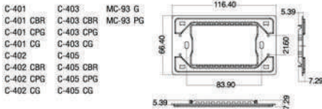
Figure 7 - ตะแกรงกดเหล็กสำหรับแผงหน้ากาก
