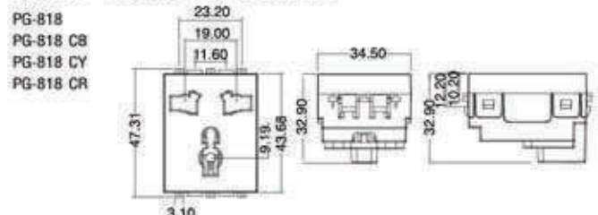
Figure 14 - เต้ารับเดี่ยวมีกราวด์ 3 ขา 18 แบบ
