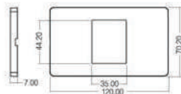
Figure 4 - แผงหน้ากราก 1 ช่องขยาย
