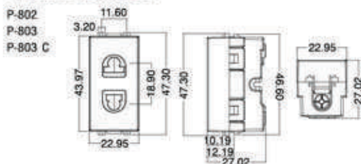
Figure 13 - เต้ารับเดี่ยว 2 ขา
