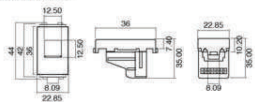
Figure 12 - ตัวรับโทรศัพท์ 6P 4C
