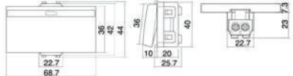
Figure 6 - สวิตช์ 2 ทางขนาดใหญ่
