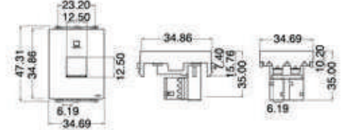
Figure 21 - เ้ารับคอมพิวเตอร์ CAT6 ขนาดกลาง
