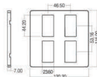
Figure 5 - แผงหน้ากรากพลาสติก 4 ช่อง
