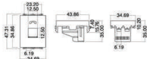
Figure 19 - เ้ารับโทรทัศน์ 6P 4C ขนาดกลาง
