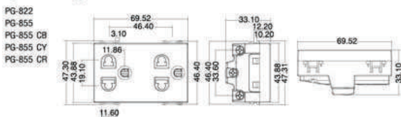
Figure 15 - เต้ารับคู่มีกราวด์ 3 ขา
