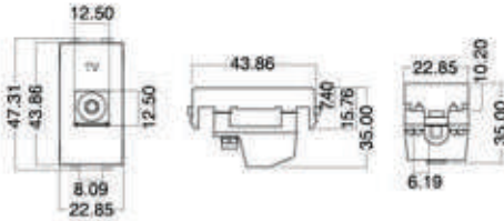
Figure 16 - เ้ารับโทรทัศน์ 75 นิ้ว ขนาดมาตรฐาน
