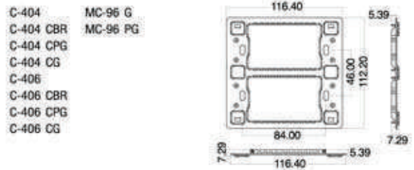
Figure 8 - ตะแกรงกดเหล็กสำหรับแผงหน้ากาก
