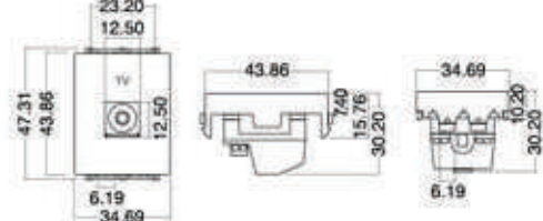
Figure 17 - เ้ารับโทรทัศน์ 75 นิ้ว ขนาดกลาง
