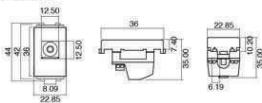
Figure 11 - ตัวรับโทรศัพท์
