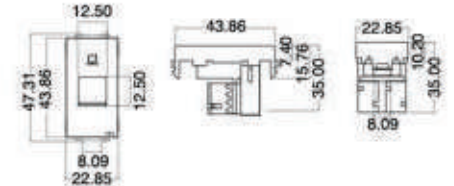
Figure 20 - เ้ารับคอมพิวเตอร์ CAT6 ขนาดมาตรฐาน
