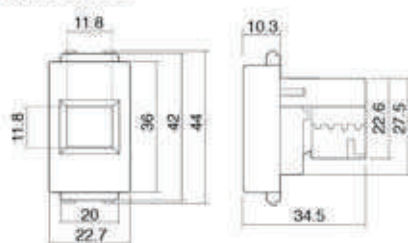
Figure 13 - ตัวรับคอมพิวเตอร์ CAT 5E
