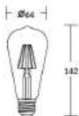
VINTAGE-V/G 4W/2700K
