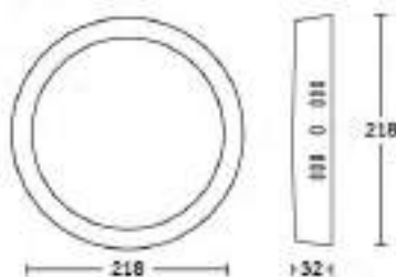
BILBO 18W
