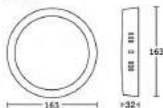
BILBO 12W
