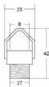
เกลียวหัวท้าย 4 พง (สามเหลี่ยม)
