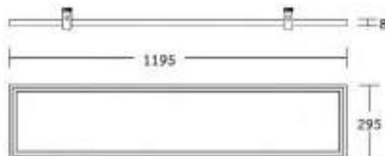
PANEL48W / 30x120
