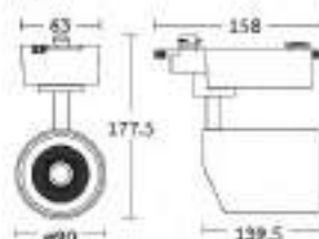
OSCAR 30W
