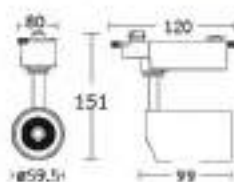
OSCAR 15W
