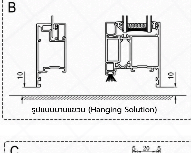
รูปแบบบานแขวน (Hanging Solution)
