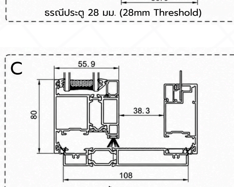
ธรณีประตู 28 มม. (28mm Threshold)
