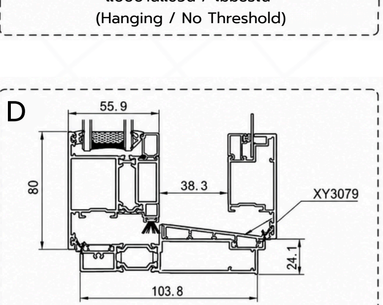
แบบบานแขวน / ไม่มีธรณี (Hanging / No Threshold)
