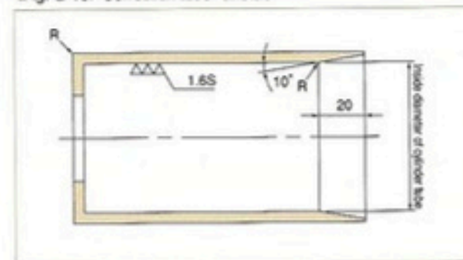
<Fig. G-18> Correction tube (metal)
