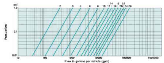
※この表は全フルボア製品についての圧力損失表であり、サイズレンジについては該当製品の範囲をご参照ください。 ※This table is for full bore products, please refer to the applicable product for the size range.
