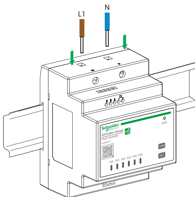
220-240V CA monofase
