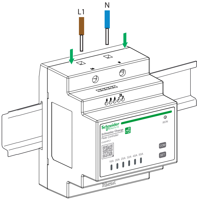
220-240V AC 1-Fase
