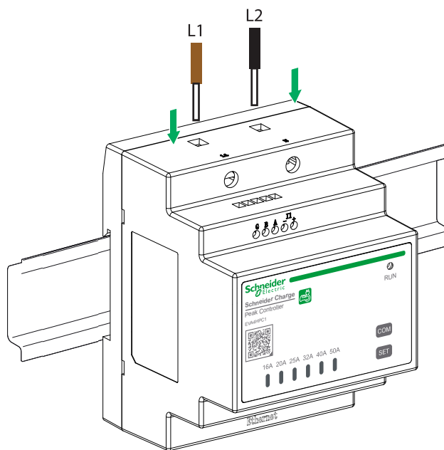
220-240V CA monofase senza neutro
