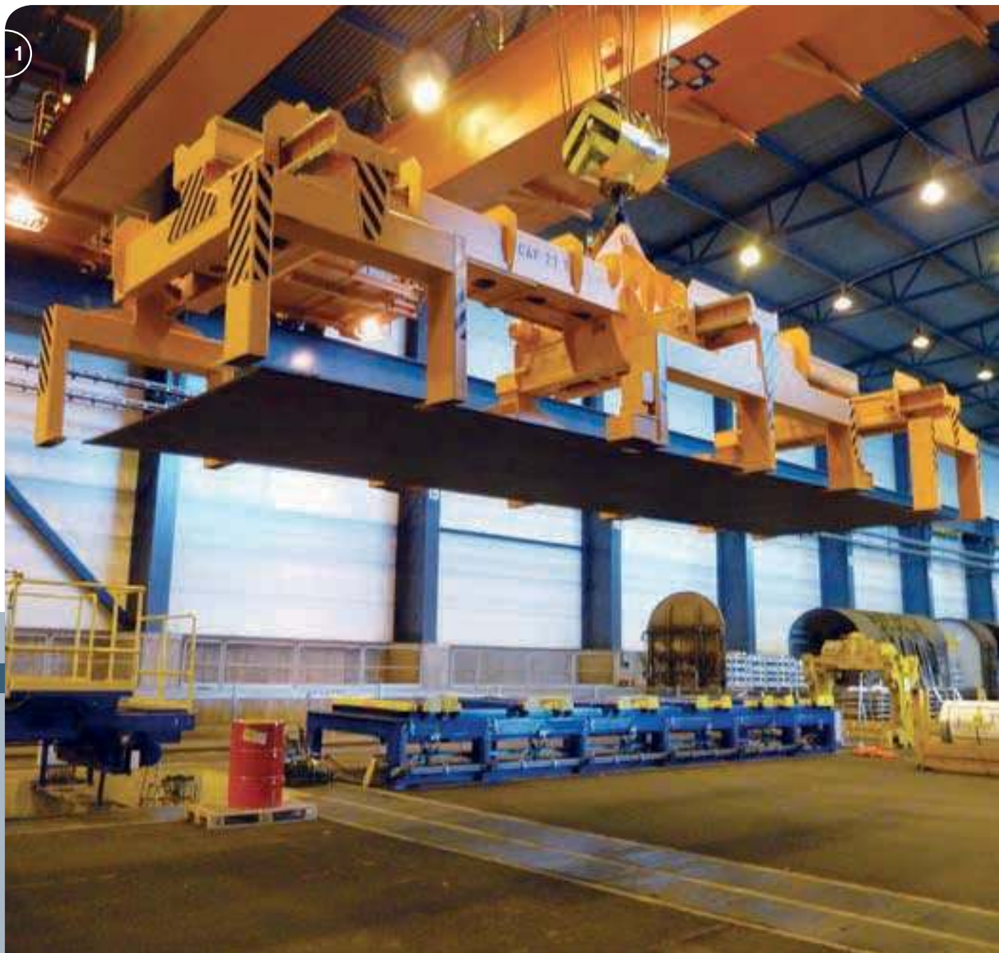
1 Elektromotorischer Blechpaketgreifer mit 27t Tragfähigkeit. Der Greifer ist in der Länge und in der Breite teleskopierbar und kann somit sehr unterschiedliche Stapel aufnehmen. Electromotive Sheet Stack Grab SWL 27t. Telescopic length and width adjustment for handling different sized stacks.
