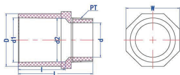
外牙直接 MALE ADAPTER (S×T)
