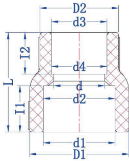
异径直接 REDUCER COUPLING (S×S)
