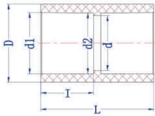
直接 COUPLING (S×S) DIN
