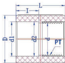
内牙直接FEMALE ADAPTER (S×T)
