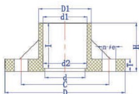
一体式法兰 FLANGE
