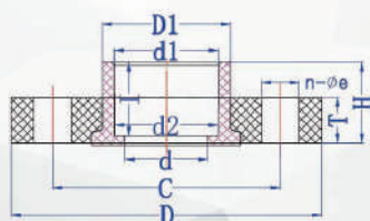
双片式法兰 VAN STONE FLANGE
