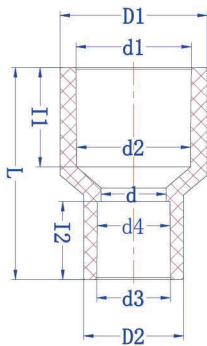
异径直接 REDUCER COUPLING (S×S) ANSI
