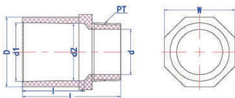
外牙直接 MALE ADAPTER (S×T)
