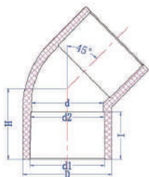
45° 弯头 45° ELBOW (S×S) ANSI
