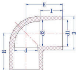
90° 弯头 90° ELBOW (S×S) ANSI
