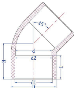
45° 弯头 45° ELBOW (S×S) ANSI
