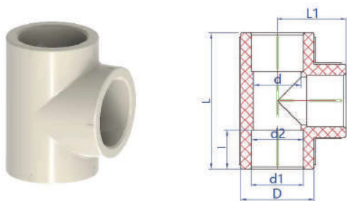
正三通 TEE (S×S)
