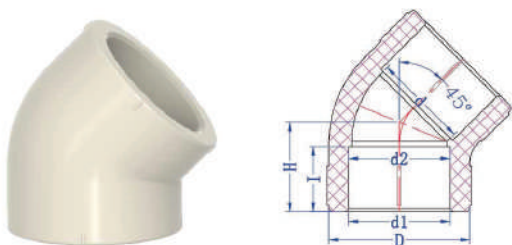
45° 弯头 45° ELBOW (S×S)
