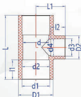
异径三通 REDUCER TEE (S×S×S) ANSI
