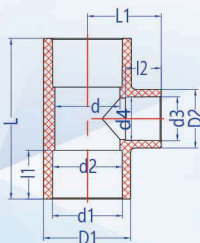
异径三通 REDUCER TEE (S×S×S) ANSI
