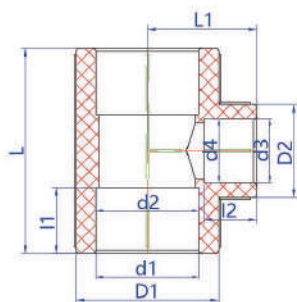
异径三通 REDUCER TEE (S×S×S)
