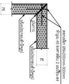
ลักษณะการต่อ "มุม 45 องศา"
