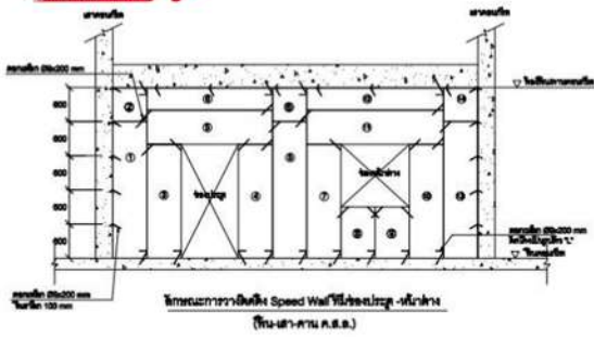
ขนาด , รูปแบบการใช้งานผนังประกอบสำเร็จรูป (Speed Wall)
