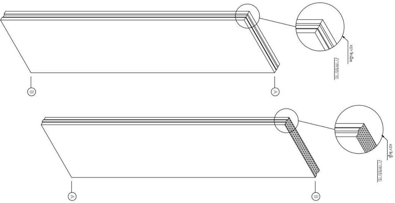
ลักษณะการติดตั้งบนพื้น/คานเหล็ก
