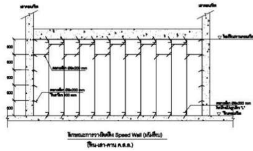
ขนาด , รูปแบบการใช้งานผนังประกอบสำเร็จรูป (Speed Wall)
