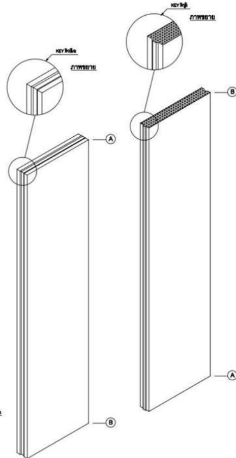
ขนาด , รูปแบบการใช้งานผนังประกอบสำเร็จรูป
