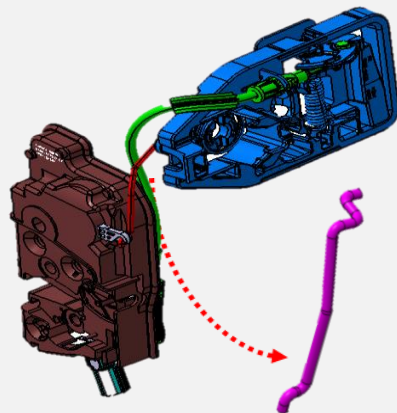
LINK ROD
