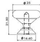
ปุ่มจับสแตนเลส STAINLESS STEEL KNOBS (PA)
