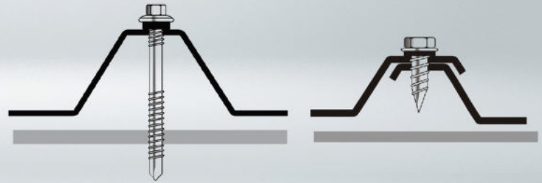
ยึดหลังคา
