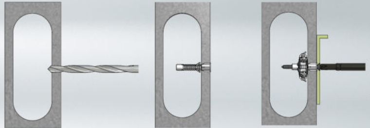
เจาะรูที่ผนังอัฐบล็อก
