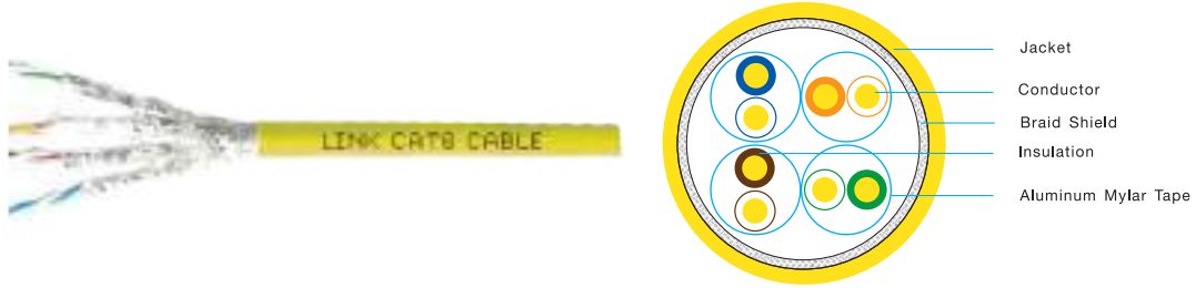
US-9488LSZH : CAT 8 S/FTP CABLE, LSZH
