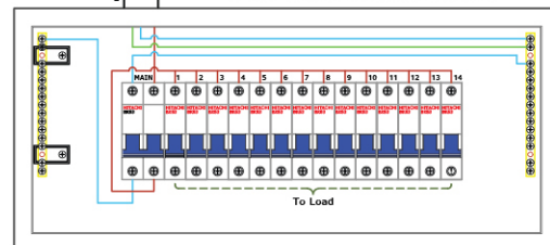
ตัวอย่างการต่อวงจรที่ไม่มีความเสี่ยงต่อไฟดูด (ไม่มีตัว RCCB ป้องกัน)
