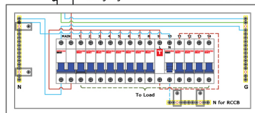
ตัวอย่างการต่อวงจรที่มีความเสี่ยงต่อกรรูกไฟดูด (ปกป้องด้วย RCCB)
