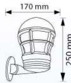
A 06-891-BK-A LAMP : E27x1 COLOR : BK MATERIAL : PLASTIC-GLASS
