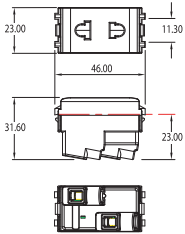
3426USM
