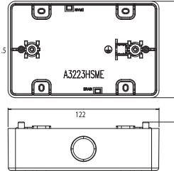
A3223HSME
