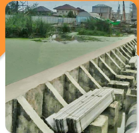
ติดตั้งแผ่นกันดินคอนกรีต
