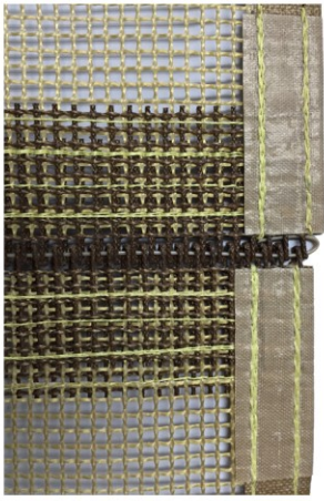
สายพานตาข่ายสำหรับเครื่องอบ UV
