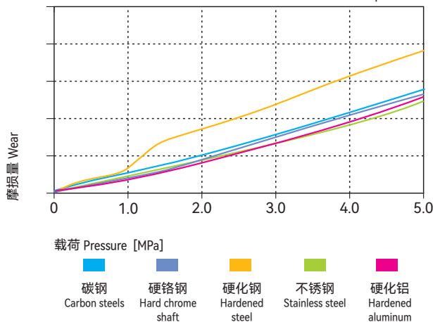
图表 Graph EPB21-8
