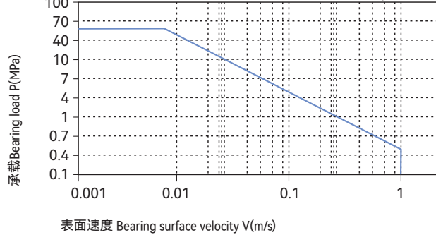
PV图表 Permissible PV value for CSB-EPB7 图表 Graph EPB7-1
