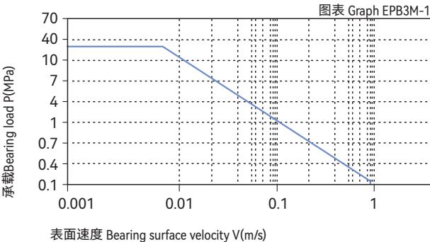
■ PV图表 Permissible PV value for CSB-EPB3M
