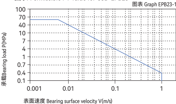
PV图表 Permissible PV value for CSB-EPB23
