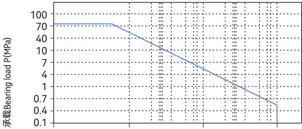
图表 Graph EPB12-1
