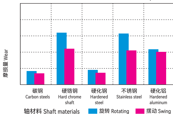
图表 Graph EPB24-7
