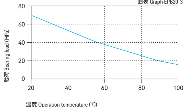
图表 Graph EPB20-3
