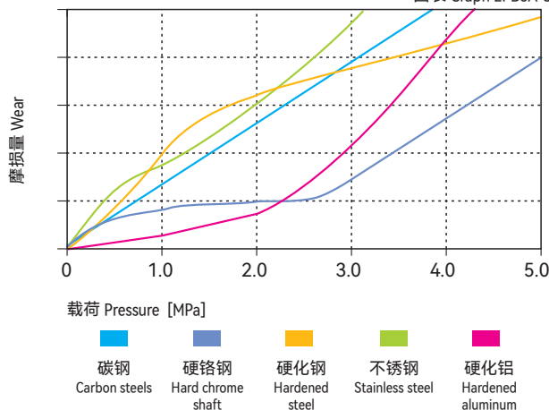
图表 Graph EPB6A-8
