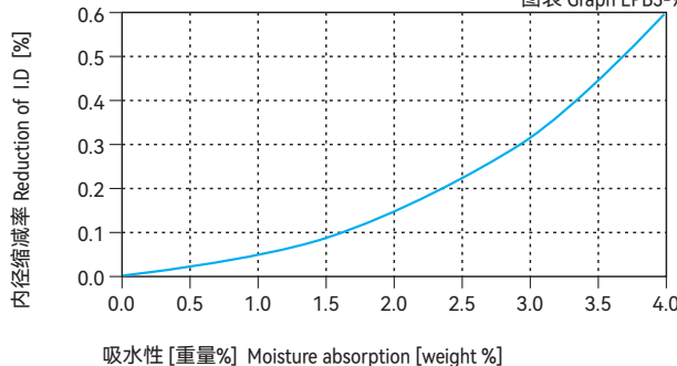
图表 Graph EPB3-9
