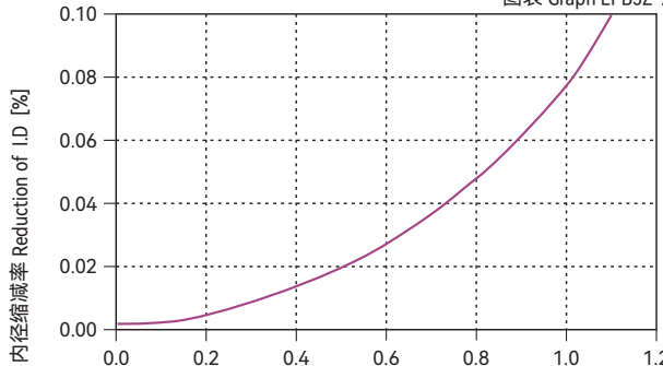
图表 Graph EPB5Z-9
