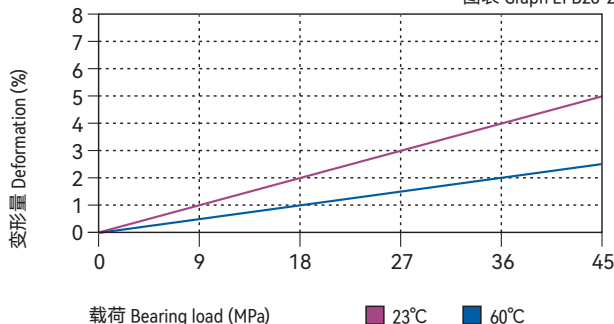
图表 Graph EPB26-2
