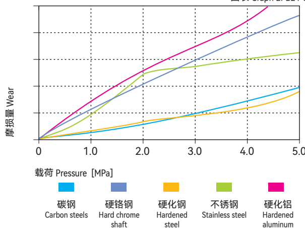
图表 Graph EPB24-8
