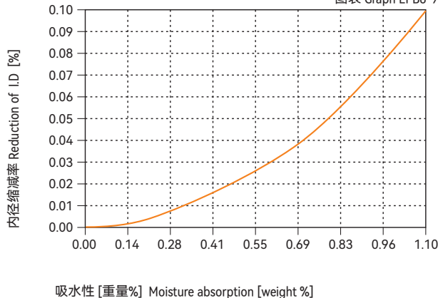
图表 Graph EPB6-9
