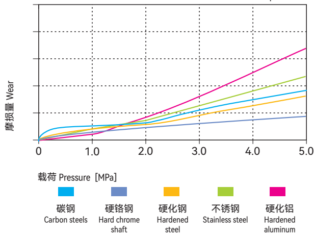
图表 Graph EPB15-8
