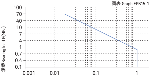
■ PV图表 Permissible PV value for CSB-EPB15
