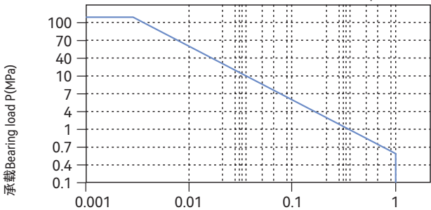
图表 Graph EPB24-1
