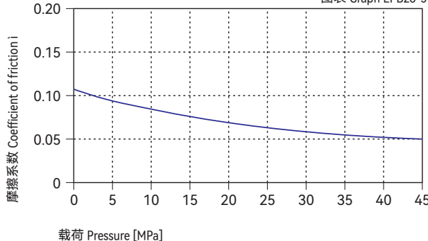
图表 Graph EPB26-5
