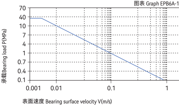
■ PV图表 Permissible PV value for CSB-EPB6A
