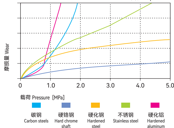
图表 Graph EPB12-8
