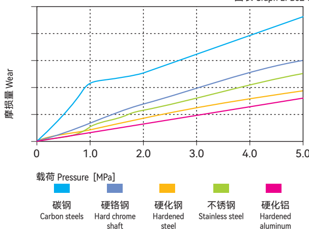
图表 Graph EPB5Z-8
