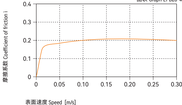
图表 Graph EPB26-4
