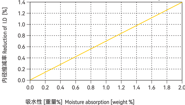
图表 Graph EPB23-9
