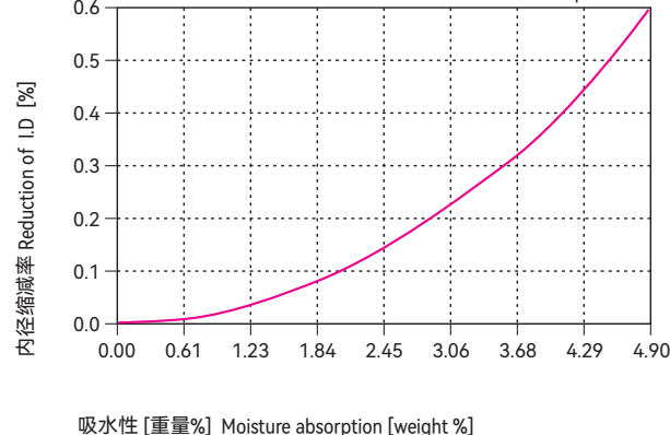
图表 Graph EPB12-9
