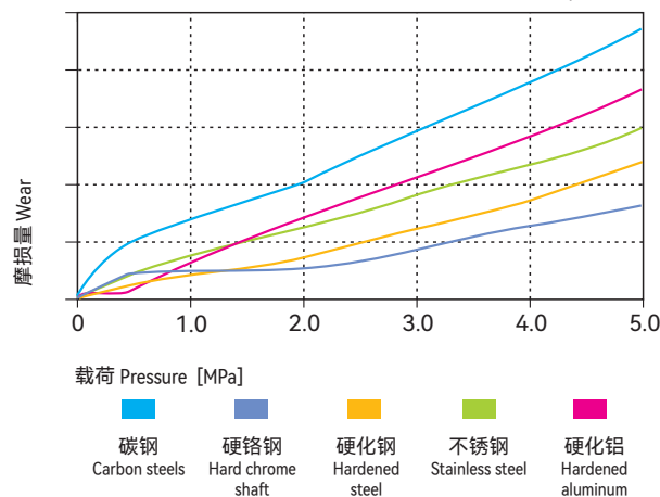
图表 Graph EPB18-8
