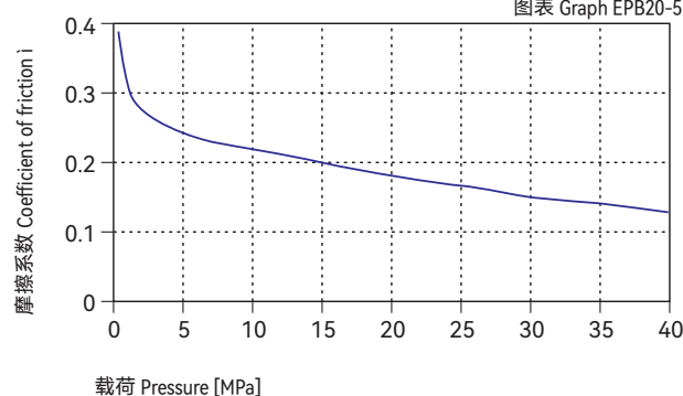
图表 Graph EPB20-5
