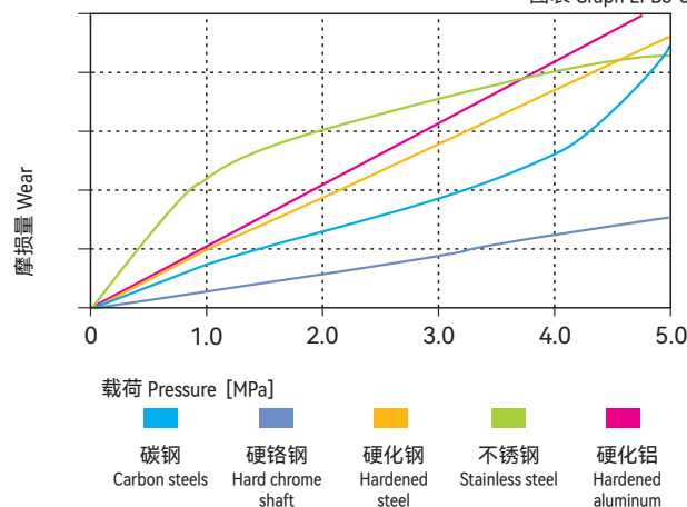
图表 Graph EPB8-8
