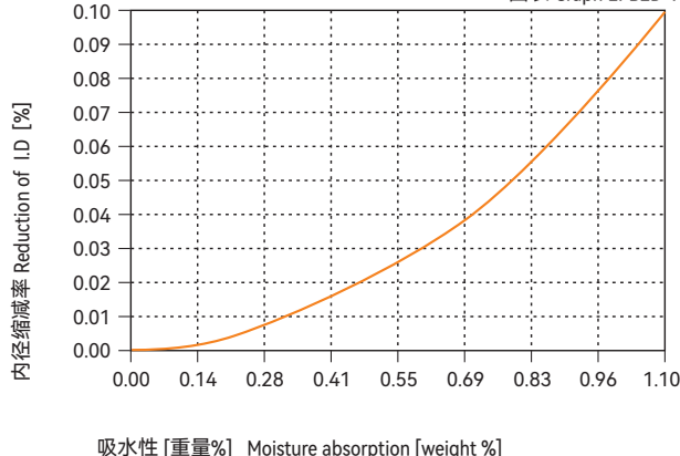
图表 Graph EPB2D-9
