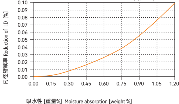
图表 Graph EPB13-9
