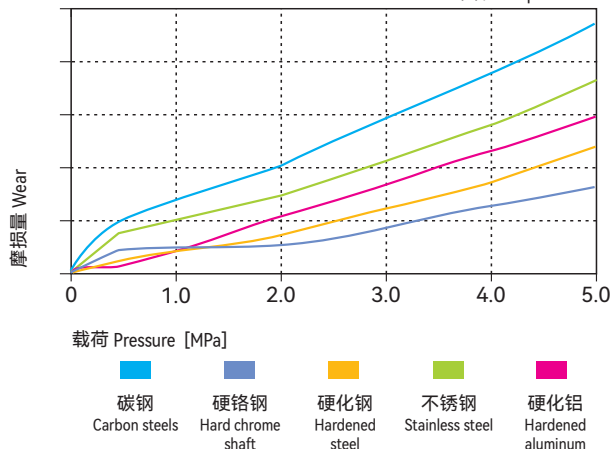
图表 Graph EPB16-8
