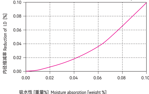
图表 Graph EPB8-9
