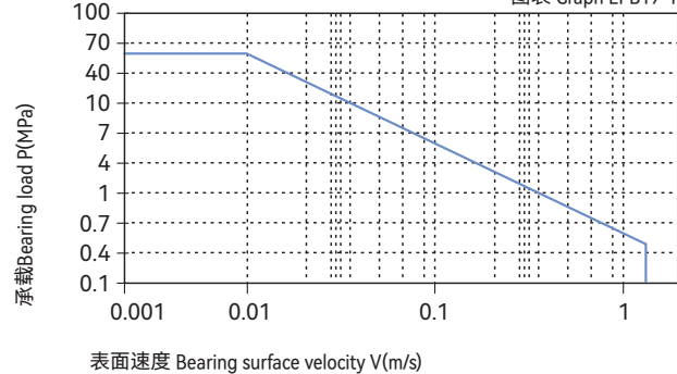
PV图表 Permissible PV value for CSB-EPB19 图表 Graph EPB19-1
