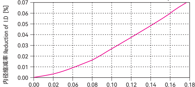
图表 Graph EPB24-9
