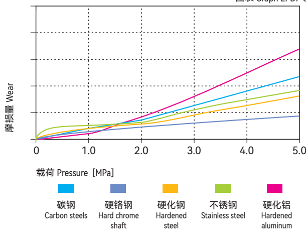
图表 Graph EPB7-8
