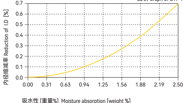
图表 Graph EPB19-9
