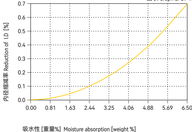
图表 Graph EPB7-9
