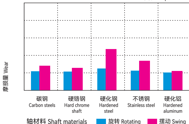
图表 Graph EPB21-7
