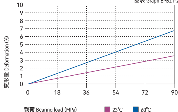
图表 Graph EPB21-2
