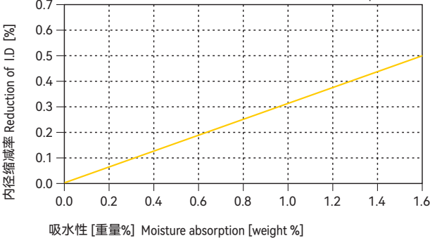
图表 Graph EPB25-9
