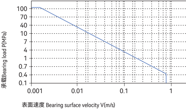
PV图表 Permissible PV value for CSB-EPB9 图表 Graph EPB9-1
