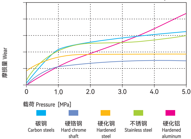
图表 Graph EPB23-8
