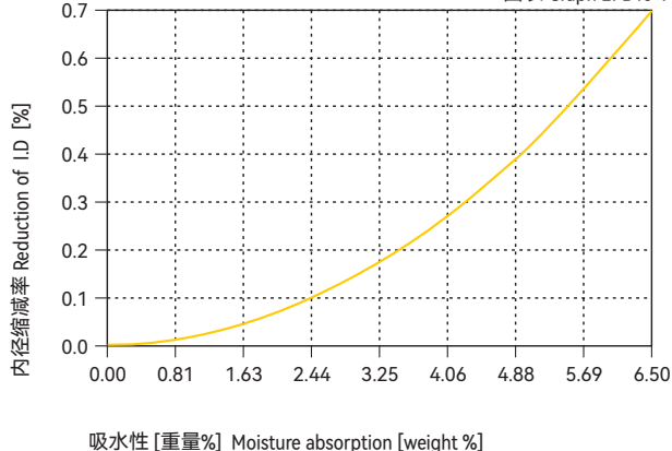
图表 Graph EPB15-9
