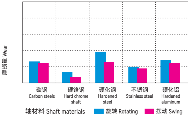
图表 Graph EPB23-7
