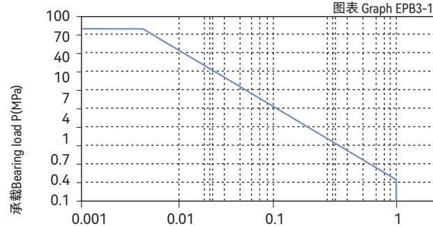
PV图表 Permissible PV value for CSB-EPB3
