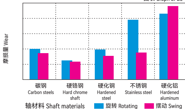
图表 Graph EPB3-7
