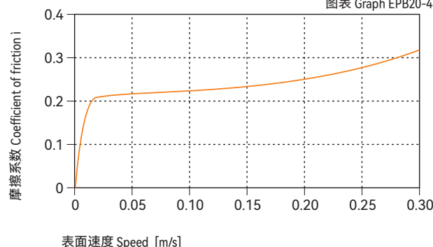
图表 Graph EPB20-4
