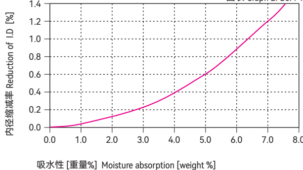
图表 Graph EPB3M-9
