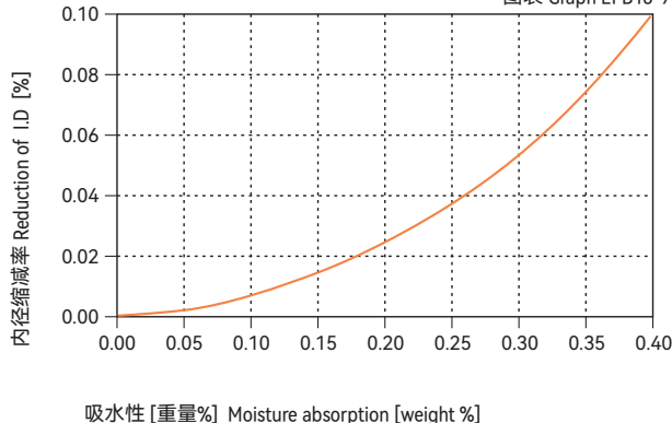
图表 Graph EPB16-9
