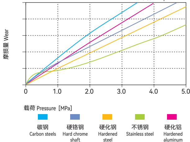
图表 Graph EPB2D-8
