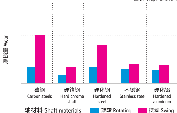
图表 Graph EPB13-7
