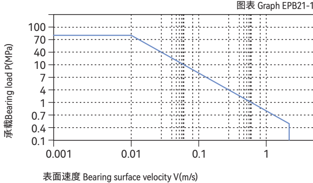
PV图表 Permissible PV value for CSB-EPB21
