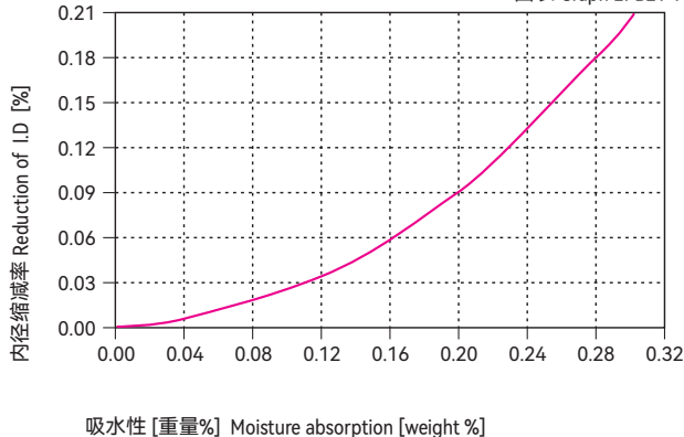
图表 Graph EPB21-9
