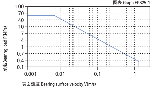
PV图表 Permissible PV value for CSB-EPB25 图表 Graph EPB25-1
