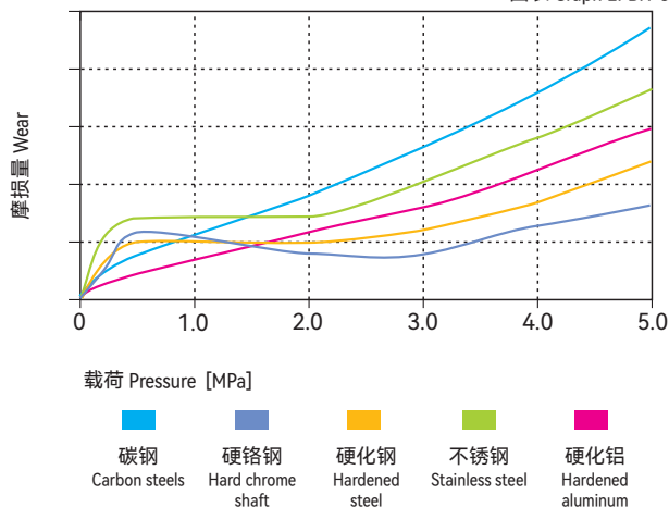
图表 Graph EPBH-8
