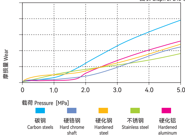
图表 Graph EPB13-8
