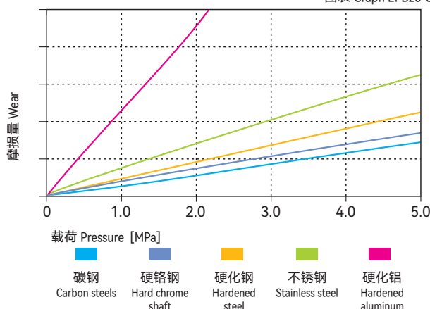
图表 Graph EPB26-8
