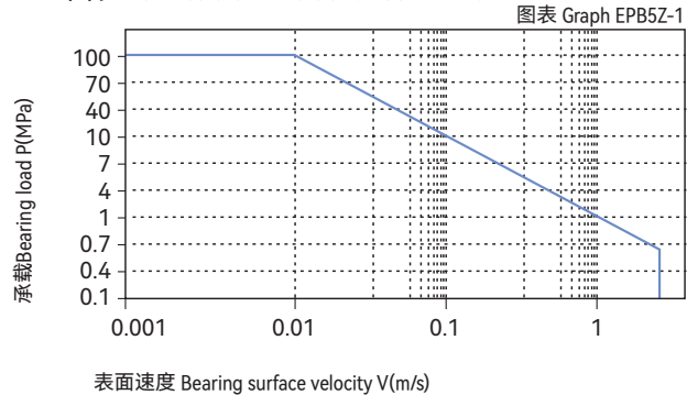
■ PV图表 Permissible PV value for CSB-EPB5Z
