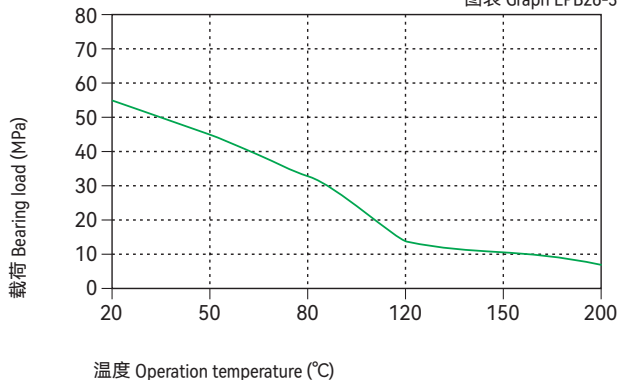
图表 Graph EPB26-3
