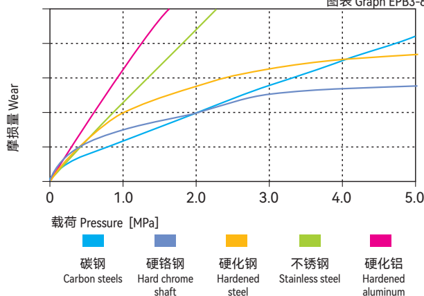
图表 Graph EPB3-8
