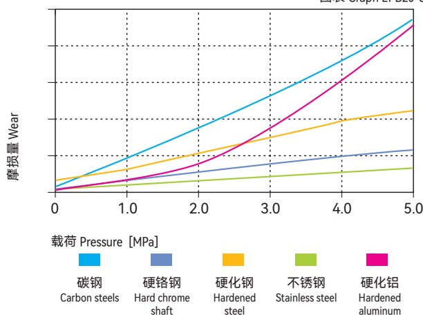
图表 Graph EPB20-8
