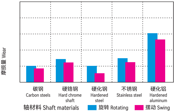
图表 Graph EPB25-7
