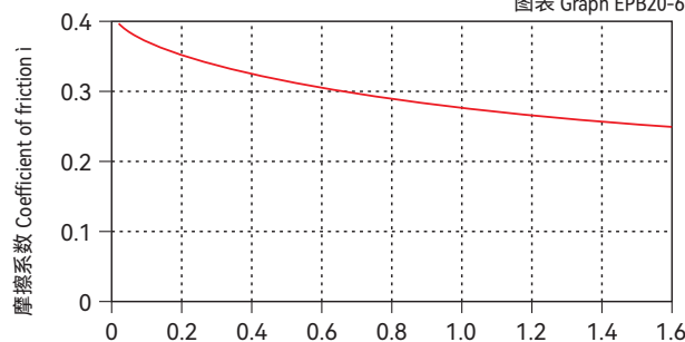
图表 Graph EPB20-6
