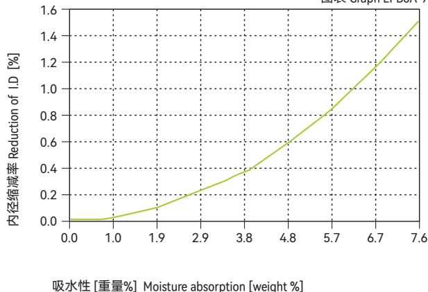
图表 Graph EPB6A-9
