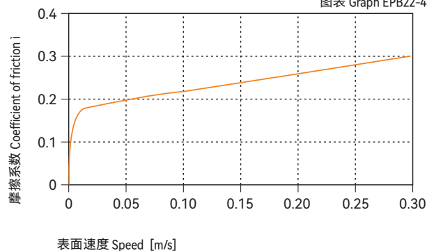
图表 Graph EPB22-4
