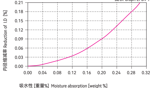
图表 Graph EPB4-9
