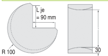
Kantenschutzwinkel mit und ohne Magnete lieferbar.
