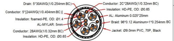
5P+4C(24AWG+28AWG)
