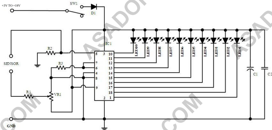
รูปที่ 1 วงจร SCHEMATIC
