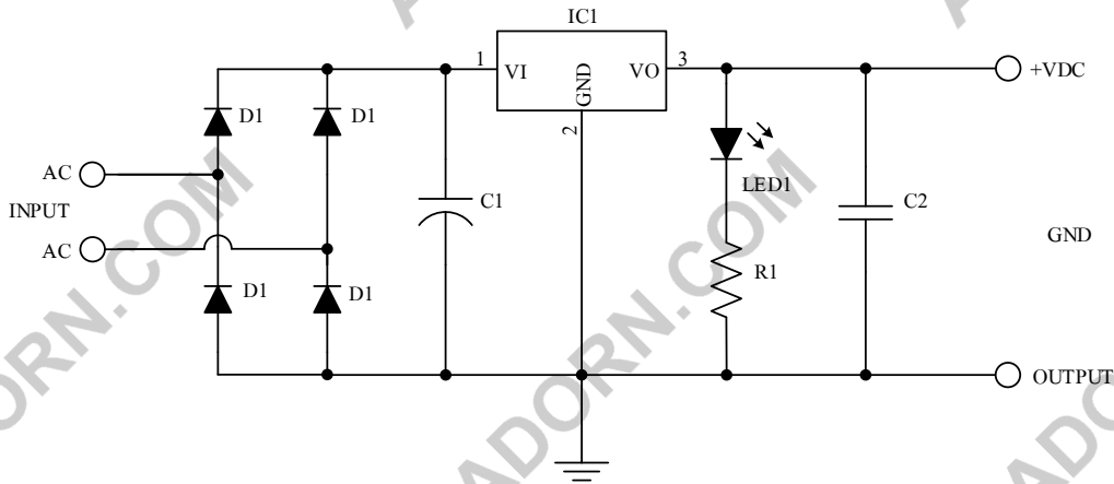
รูปที่ 1 วงจร SCHEMATIC
