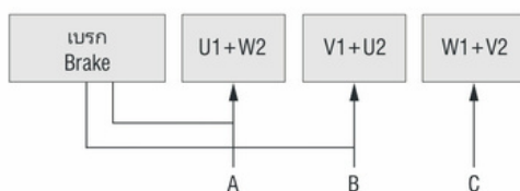
Δวิธีการเชื่อมต่อ/220V-240V
