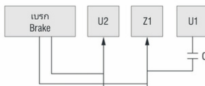
100W/200Wการเชื่อมต่อหวนเข็มนาฬิกา/CCW Connection
