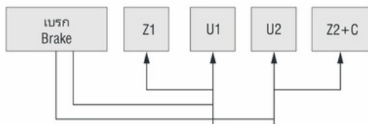
400W/750Wการเชื่อมต่อตามเข็มนาฬิกา/CW Connection
