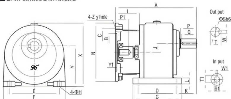
■ ZHM แนวนอน ZHM Horizontal
