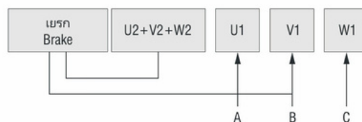
Yวิธีการเชื่อมต่อ/380V-415V
