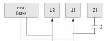
100W/200Wการเชื่อมต่อตามเข็มนาฬิกา/CW Connection
