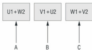
Δวิธีการเชื่อมต่อ/220V-240V
