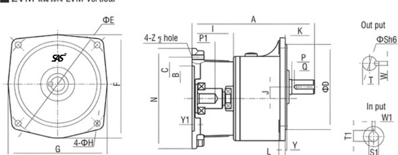
■ ZVM แนวตั้ง ZVM Vertical
