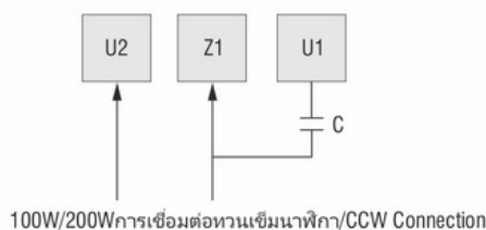
100W/200Wการเชื่อมต่อหวนเข็มนาฬิกา/CCW Connection
