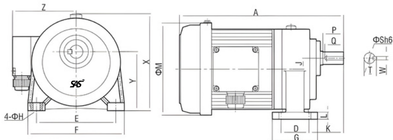
■ แนวนอน Horizontal
