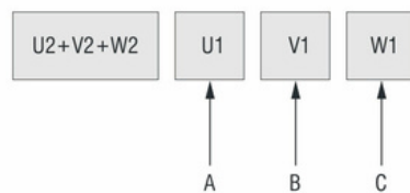
Y วิธีการเชื่อมต่อ/380V-415V
