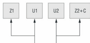
400W/750W/1500Wการเชื่อมต่อตามเข็มนาฬิกา/CW Connection
