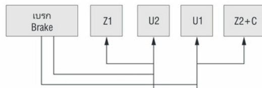
400W/750Wการเชื่อมต่อหวนเข็มนาฬิกา/CCW Connection
