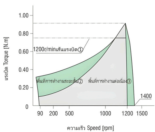
● 5IK120RGU-CF (220V/50Hz) (ZD ตัวขับเคลื่อนมาตรฐาน ZD standard drive)
