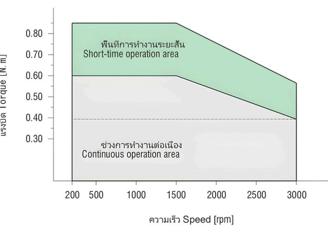
● Z5BLD120-220GU-30S กราฟเส้น Diagram (ZD ตัวขับเคลื่อนมาตรฐาน ZD standard drive)
