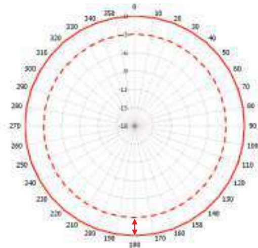
รูปที่ 2 แสดงแบบรูปกำลังของสายอากาศรับสัญญาณภายในอาคารแบบแอกทีฟ แบบที่ 2
