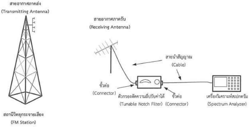
รูปที่ 2 ฝั่งการต่อเครื่องมือสำหรับการทดสอบการแพร่แปลงปลอมผ่านสายอากาศ
